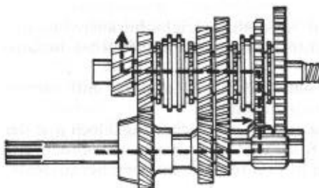
Bild G 7. Kraftverlauf für den Rückwärtsgang
