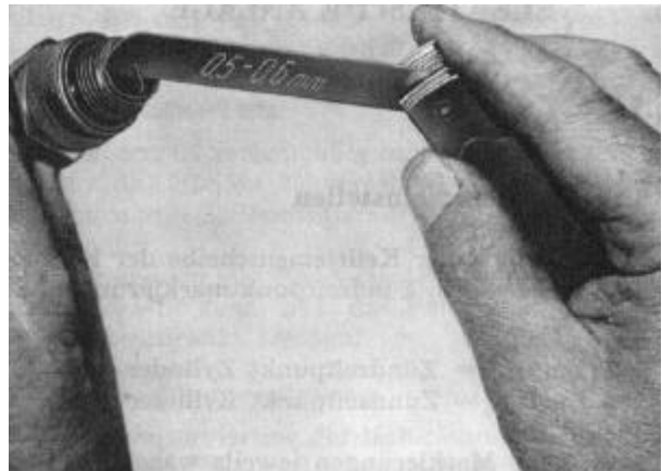
Bild E 4. Elektrodenabstand überprüfen
