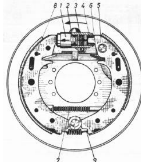
Bild F 40. Radbremse hinten
