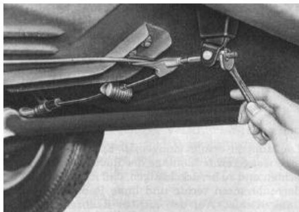
Bild F 54. Handbremse nachstellen
