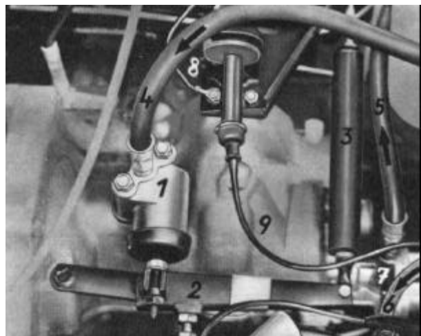
Bild H 16. Aggregate am Getriebe
