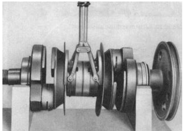
Bild M 31. Flachschiebergabel einsetzen
