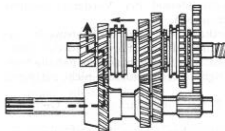
Bild G 6. Kraftverlauf für den 4. Gang
